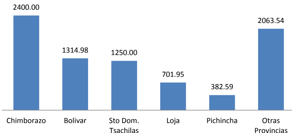
SUPERFICIE FORESTADA Y REFORESTADA CON ESPECIES NATIVAS POR GAD PROVINCIAL 2016 (ha)
