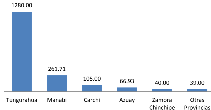
SUPERFICIE FORESTADA Y REFORESTADA CON ESPECIES ADAPTADAS/INTRODUCIDAS POR GAD PROVINCIAL 2016 (ha)
