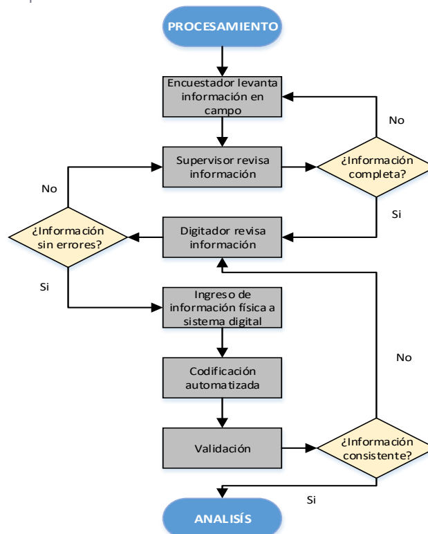
Gráfico 3. Flujograma procesamiento.
